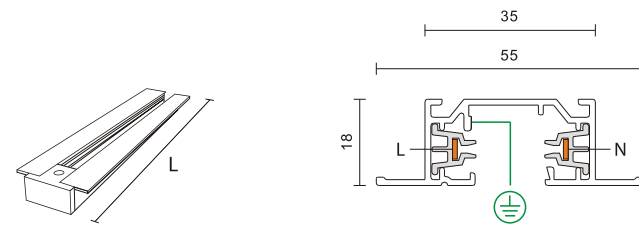
HTC-1M、2M、3M 1-Circuit Track(Recessed) 220V, 16A
