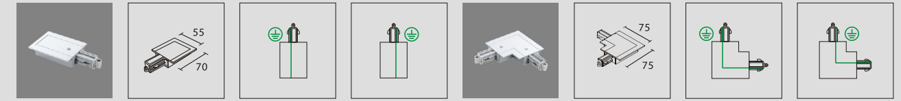
HTC-L01(L/R) Live end 230V, 16A
